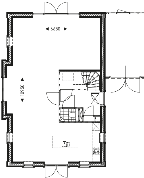
BEGANE GROND
