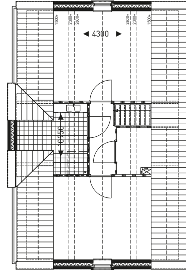
2E VERDIEPING
