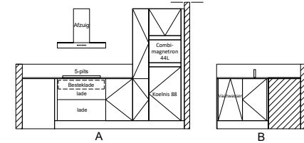
Aanzichten Keuken
