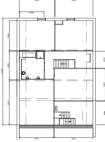
verdieping
