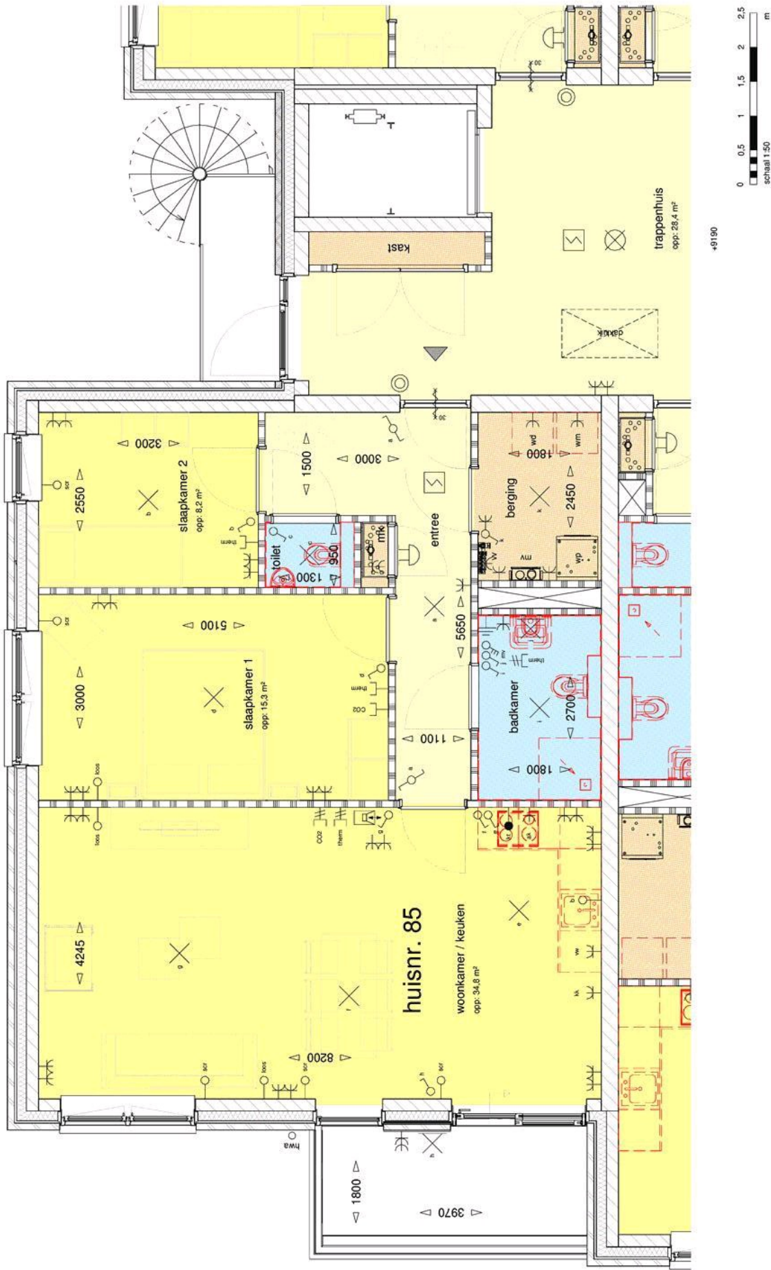
1866 02-12-2020 nieuwbouw 2 appartementengebouwen Hutten Zuid te Ulfst 3e verdieping - huisnummer 85
